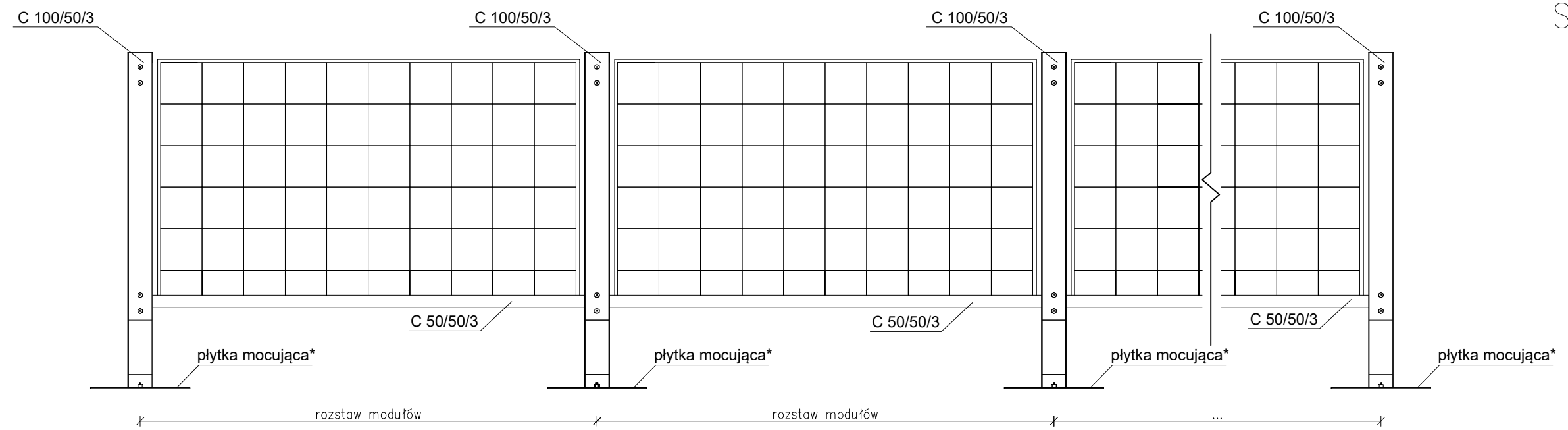
WIDOK Z PRZODU SKALA 1:20
